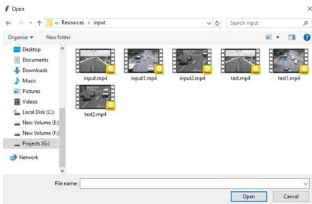
Fig.2. Input video.
